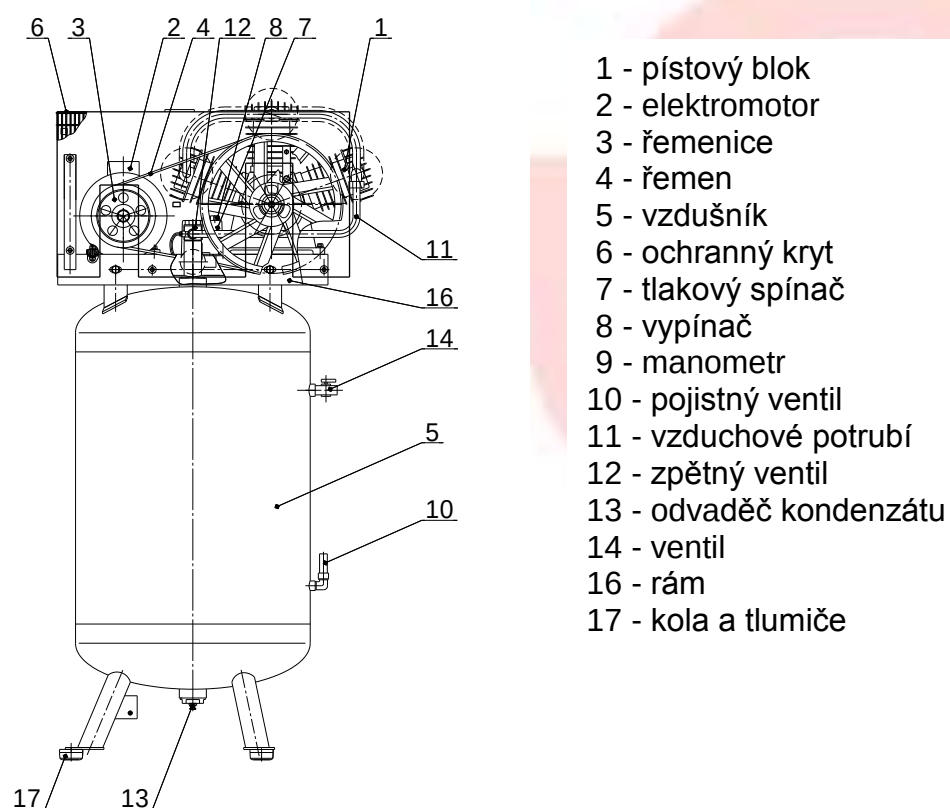
Obr. 9 - Celkový pohled na kompresor F-270.LB40B
