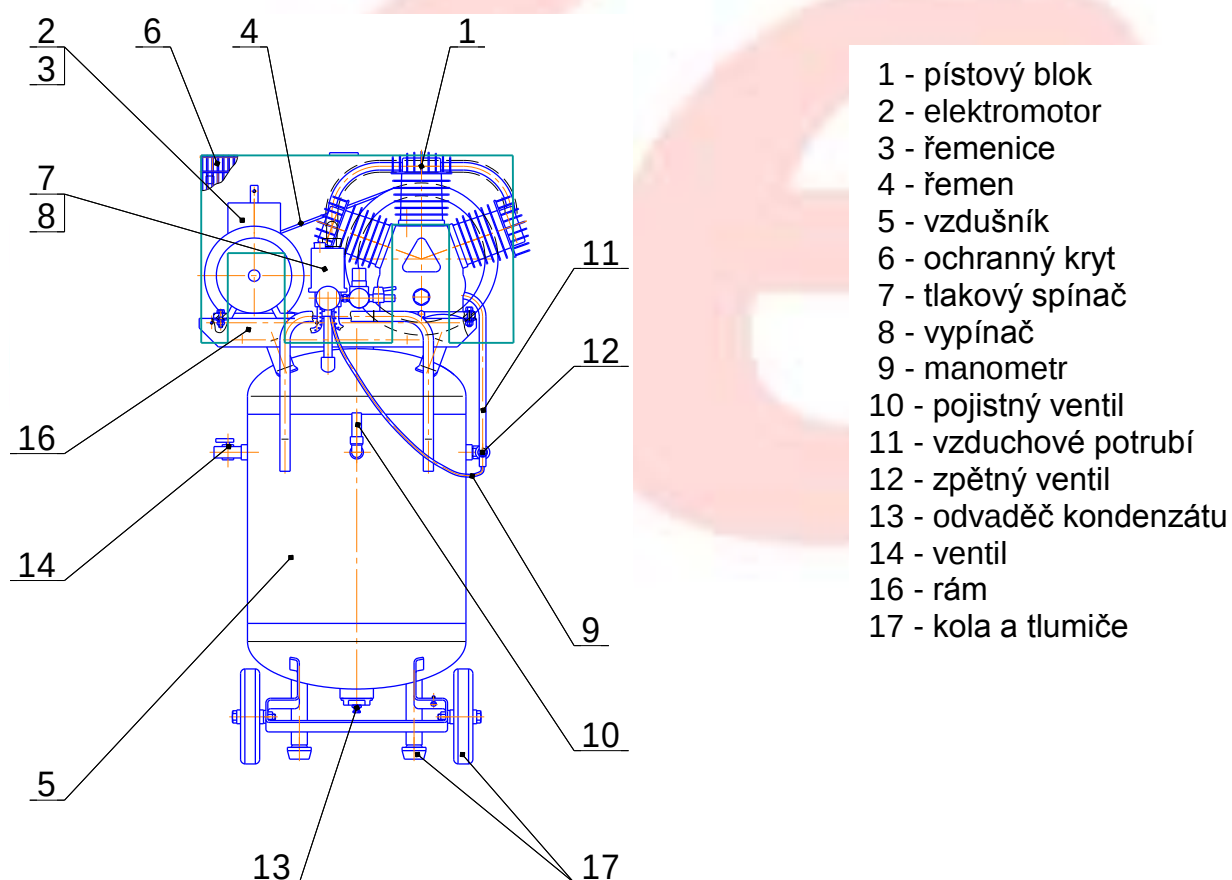
Obr. 7 - Celkový pohled na kompresor C-100.LB40B
