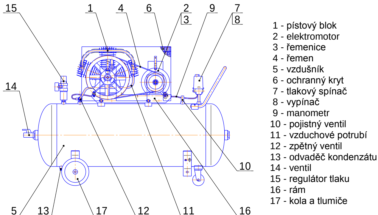
Obr. 8 - Celkový pohled na kompresor C-200.LB40
