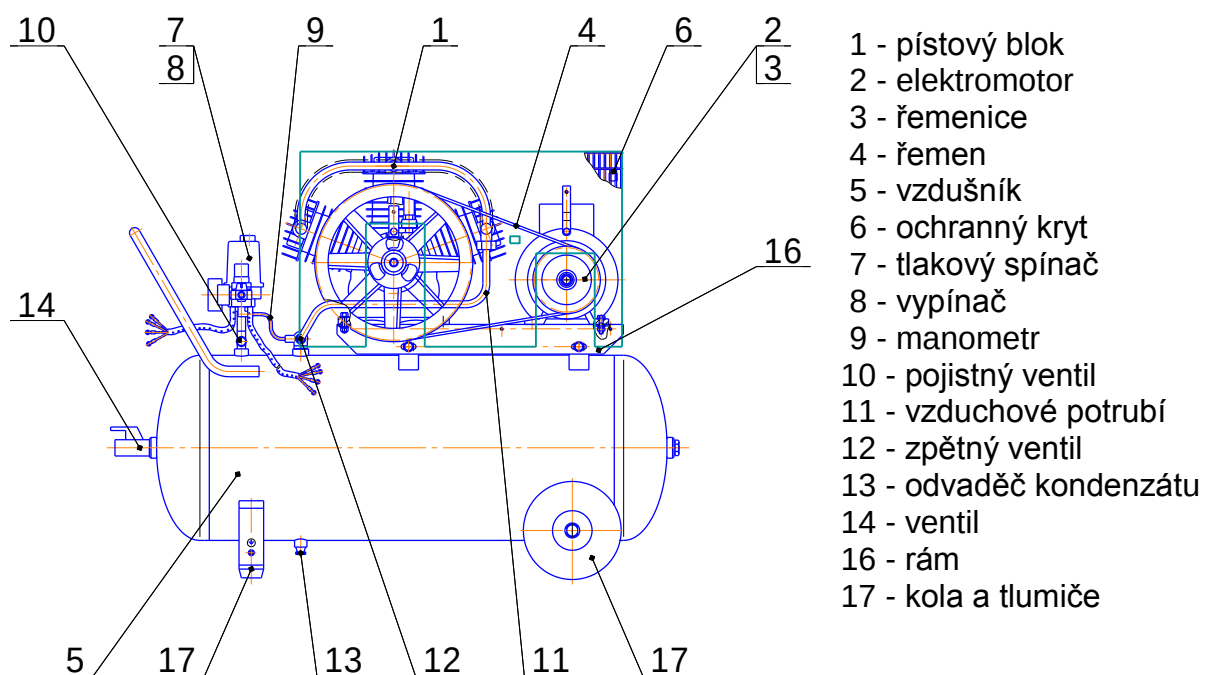
Obr. 6 - Celkový pohled na kompresor C-100.LB40
